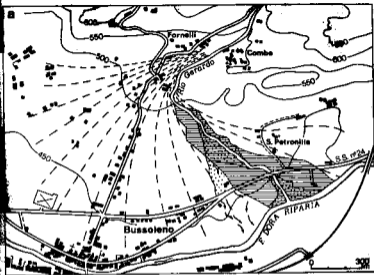
Fig. 27 - Conoide alluvionale del T. Gerardo in Comune di Bussoleno (Valle di Susa). Il settore sinistro del conoide è ricorrentemente soggetto a inondazioni e alluvionamenti. In (a): 1) area complessivamente interessata dagli eventi del maggio 1947, agosto 1972, giugno 1973; 2) idem, giugno 1957. In (b): 3) area alluvionata nel maggio 1977. Le frecce indicano la direzione delle correnti di esondazione (da Mortara e Tropeano, 1978, modificato).
