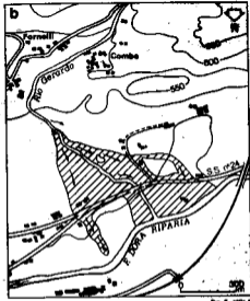
Fig. 27 - Conoide alluvionale del T. Gerardo in Comune di Bussoleno (Valle di Susa). Il settore sinistro del conoide è ricorrentemente soggetto a inondazioni e alluvionamenti. In (a): 1) area complessivamente interessata dagli eventi del maggio 1947, agosto 1972, giugno 1973; 2) idem, giugno 1957. In (b): 3) area alluvionata nel maggio 1977. Le frecce indicano la direzione delle correnti di esondazione (da Mortara e Tropeano, 1978, modificato).
