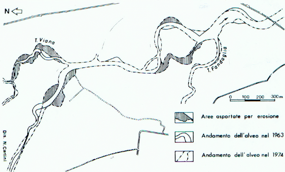
FIG. 14 - Planimetria del T. Malone nel tronco compreso tra la confluenza dei torrenti Viana e Fandaglia, ove gli effetti della piena del giugno '73 furono maggiormente sensibili.
